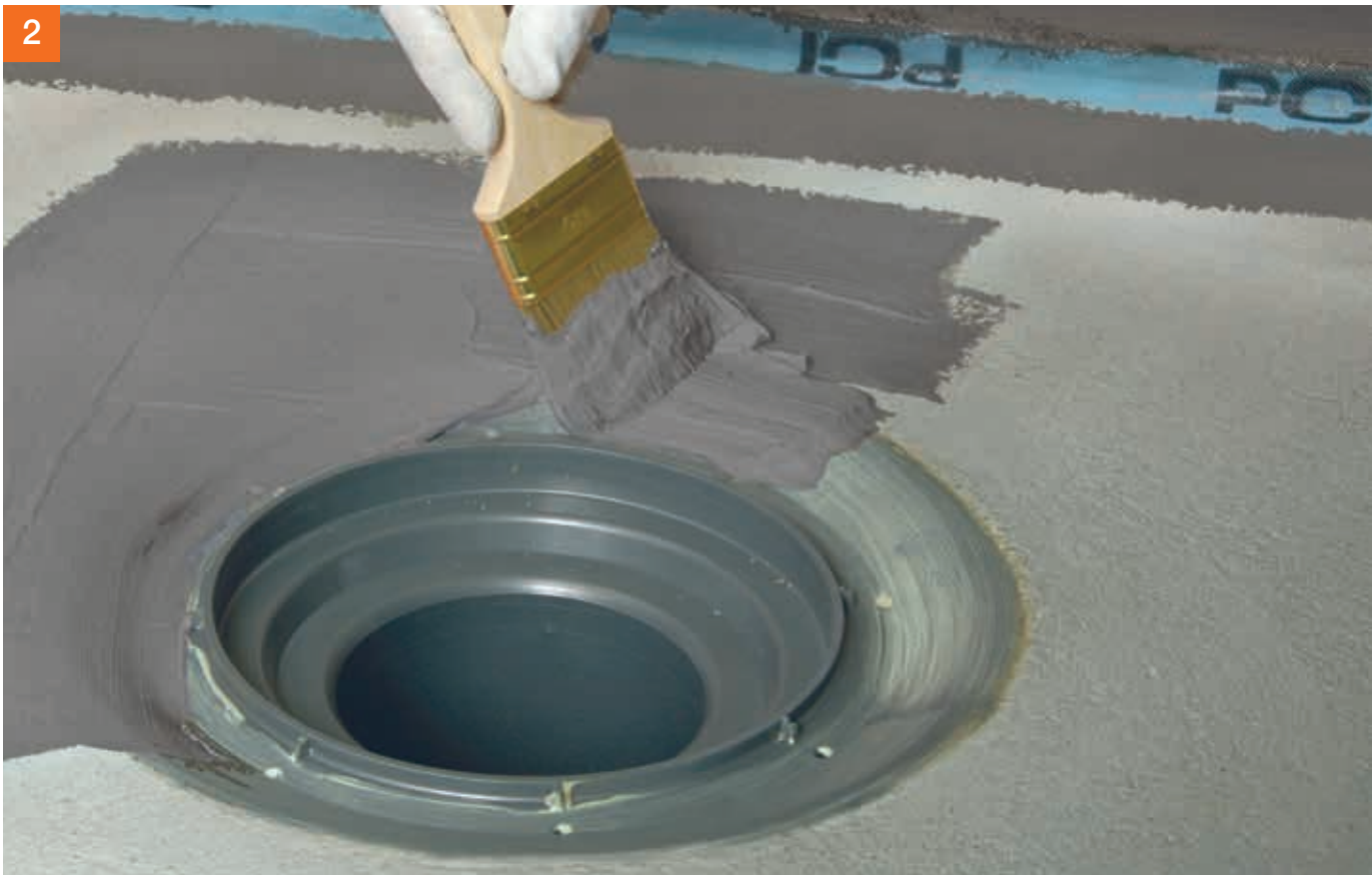
PCI Seccoral® 1K / 2K Rapid vorlegen ...
