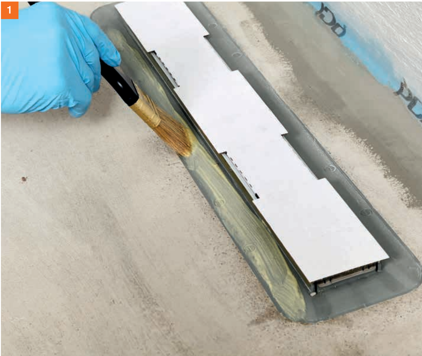
Grundierung des Anschlussflansches mit PCI Epoxigrund.
