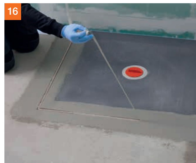
... Klebestreifen abziehen ...
