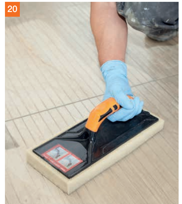
... waschen und sauber abziehen.
