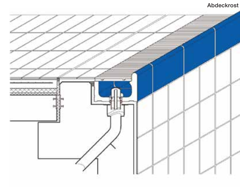
System Wiesbaden, hochliegend: Großer Rinnenstein mit Handfasse, Abdeckrost und Flüsterablauf SILENT W 2000. Für vielfältige Bäderarten verwendbar.
