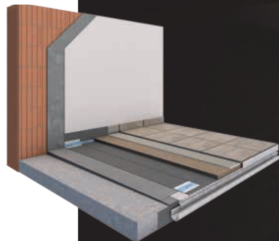
System II Balkon / Terrasse
