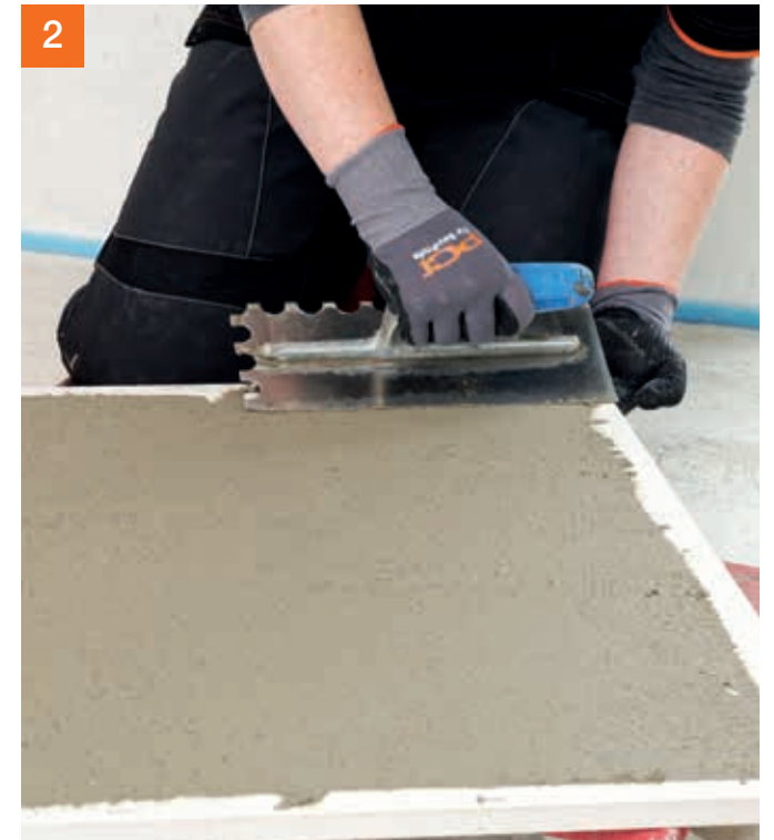
2 Aufbringen der rückseitigen Kratzspachtelung, um eine nahezu hohlraumfreie Verlegung zu gewährleisten.
