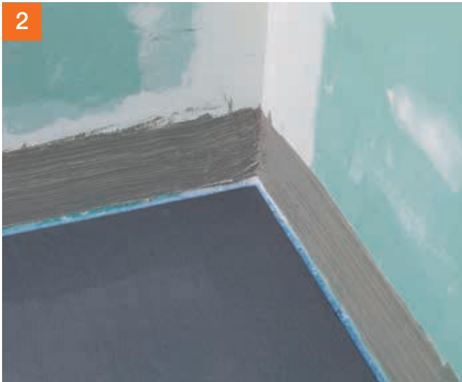
Anschließend wird zum Verkleben des Sicherheits-Dichtbands PCI Pecitape® 120 das Abdichtungsmaterial PCI Seccoral® 1K / 2K Rapid an der Wand vorgelegt.
