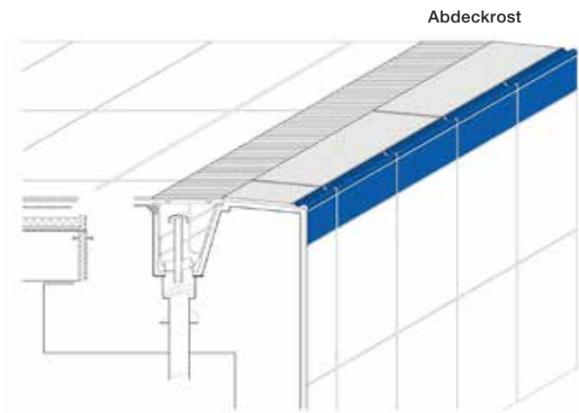
System Finnland II: Schräger, strandähnlicher Beckenrand mit Handfasse, abgedeckte Rinne mit Rinnenschale und Flüsterablauf SILENT 100. Besonders geeignet für Sport- und Wettkampfbecken.
