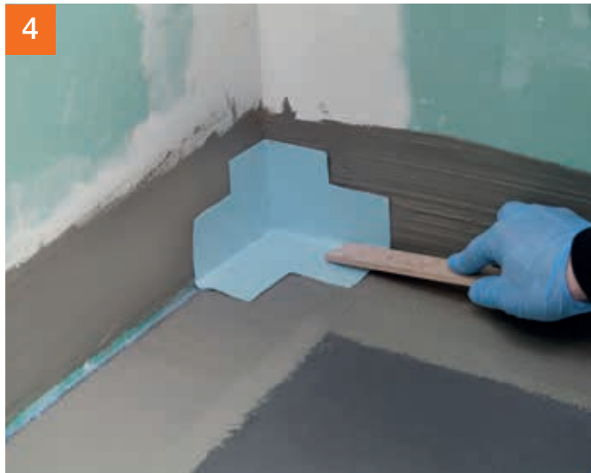
Einlegen der vorgefertigten Spezial-Innenecke PCI Pecitape® 90° L in PCI Seccoral® 1K / 2K Rapid.
