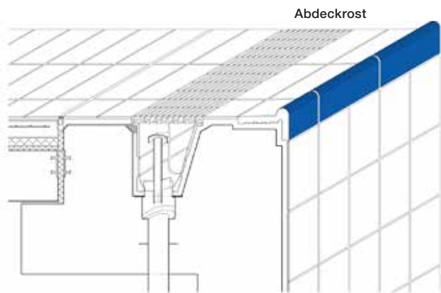
System Zürich: Hochliegende Überflutungskante als Handfasse, abgedeckte Rinne mit Rinnenschale und Flüsterablauf SILENT 100. Für öffentliche Bäder.
