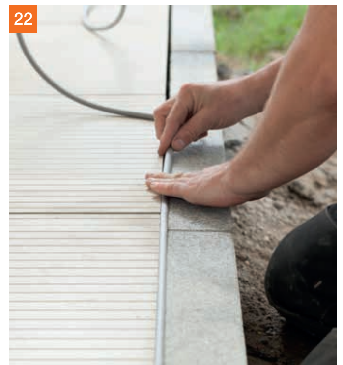
Danach die Rundschnüre einbauen für das nachfolgende Silikonieren.
