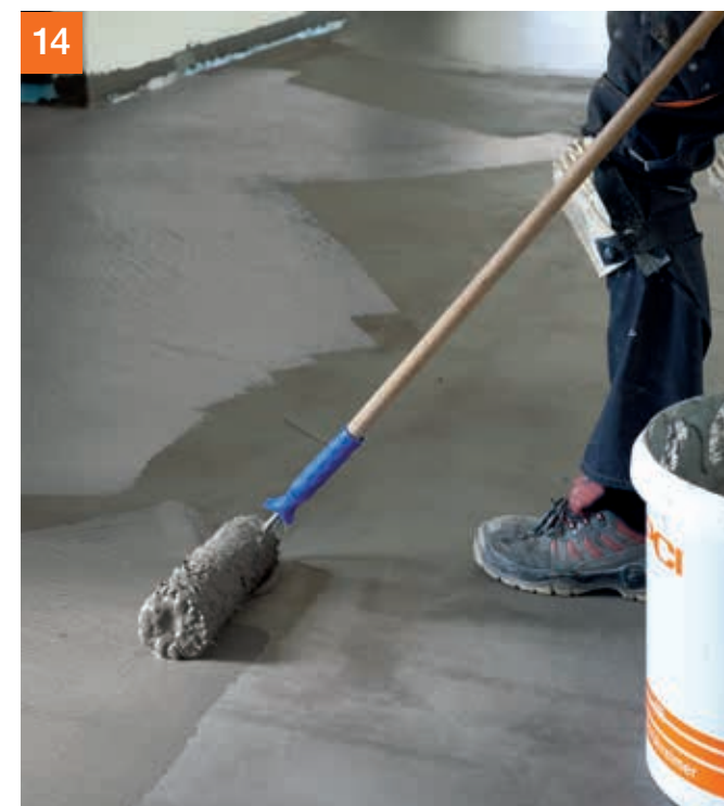
PCI Seccoral® 2K Rapid kann auch – bis zum Erreichen der erforderlichen Trockenschichtdicke von 2 mm – mittels Lammfellrolle aufgetragen werden.
