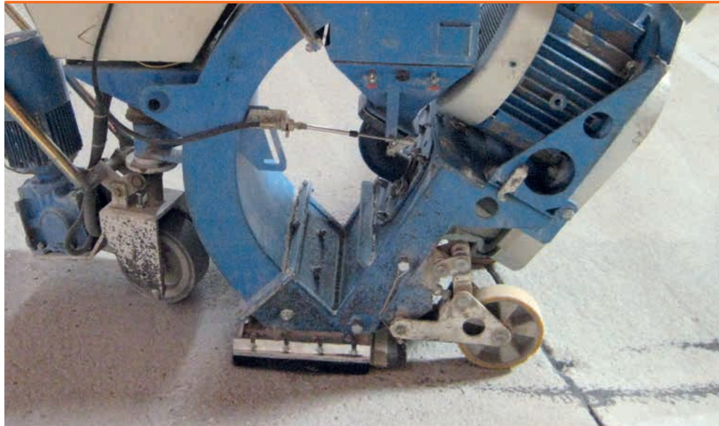
Kugelstrahlgerät
