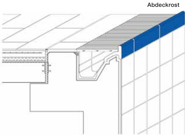
System Berlin: Hochliegende Überflutungskante als Handfasse, abgedeckte Rinne mit „weichem“ Einlauf. Für öffentliche Bäder und Sanierungen.
