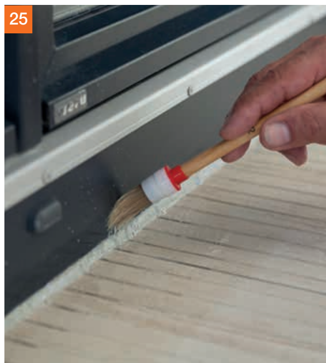
25 Zum leichteren Abziehen der Silikofuge zum Beispiel PCI Glättmittel auftragen ...
