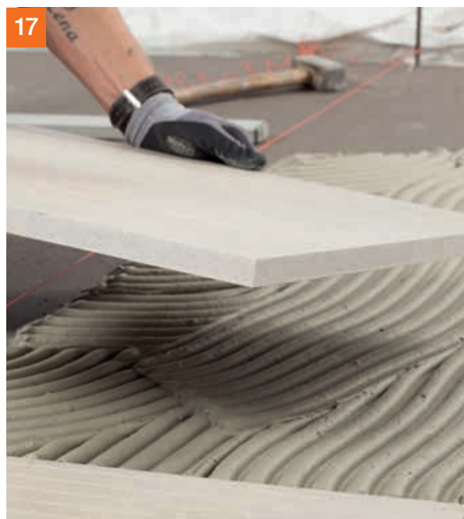
... Fliese einlegen ...
